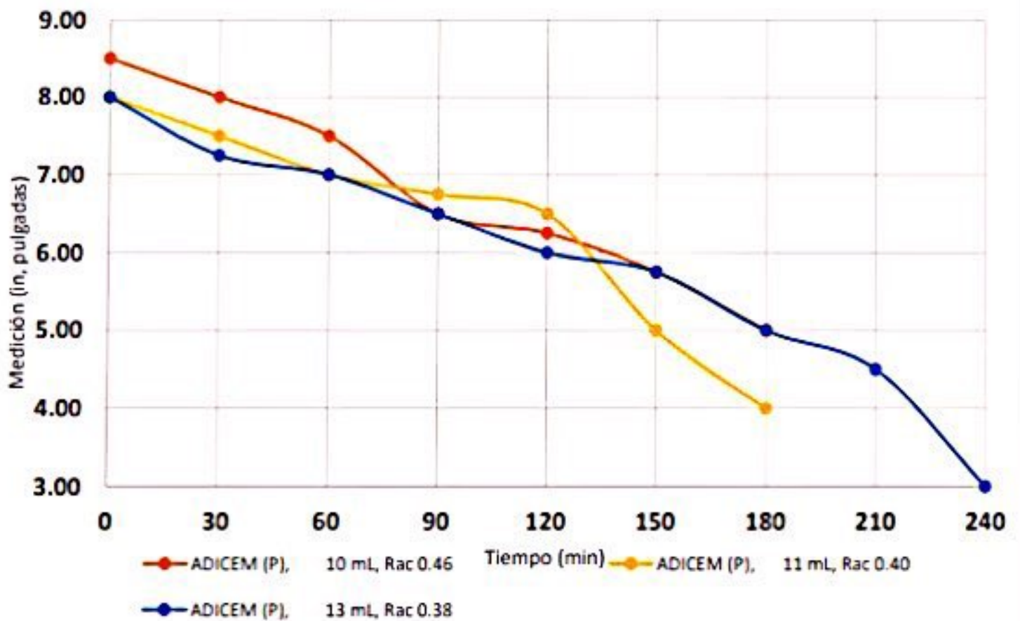
Desarrollo de trabajabilidad de mezclas utilizando aditivo ADICEM con diferentes relaciones AC
