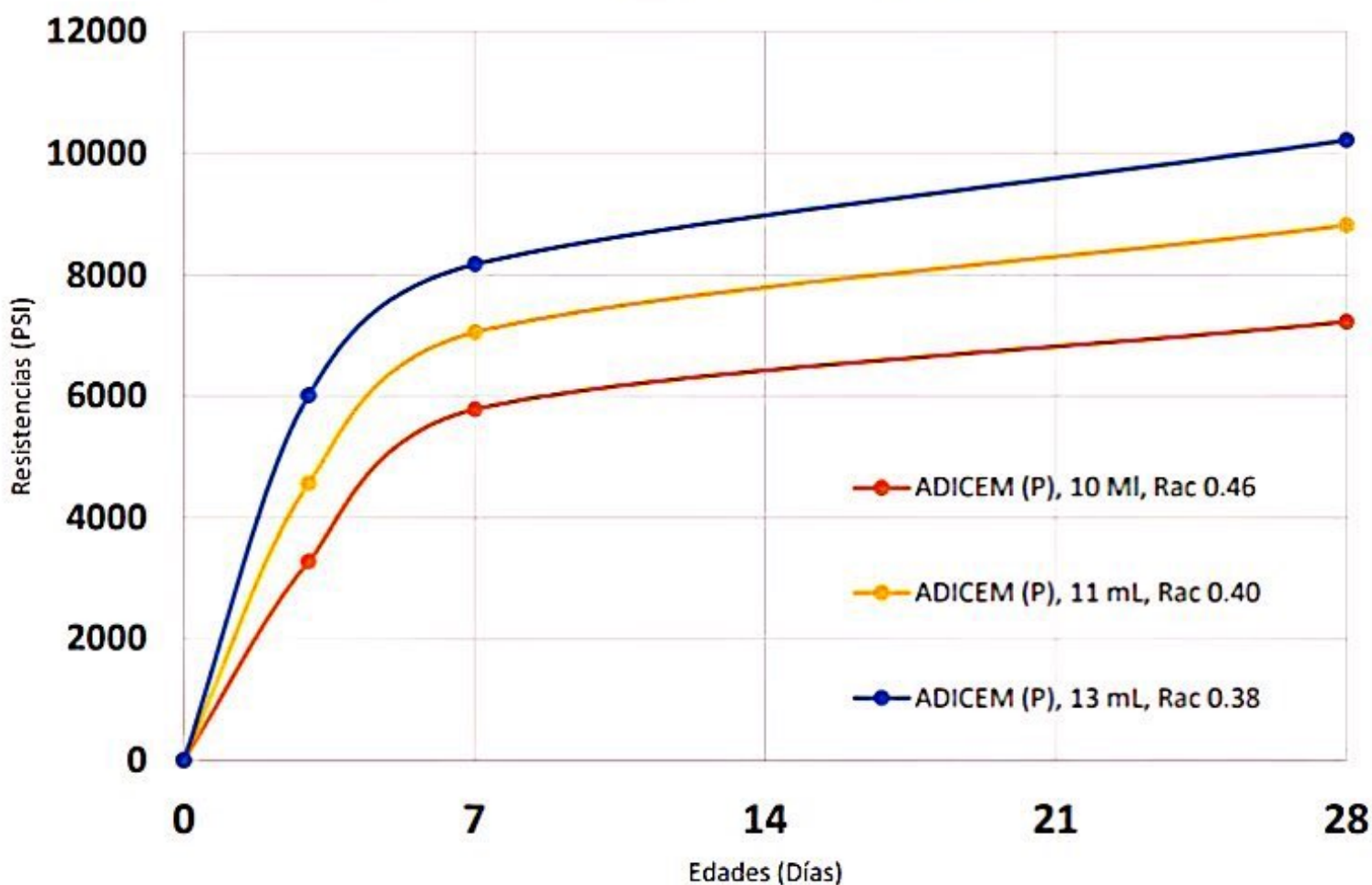
Desarrollo de resistencias de aditivos para proyecto Panamá
